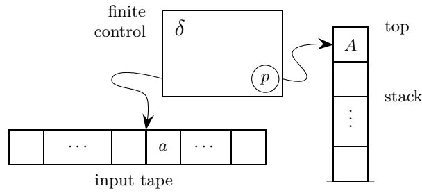
Fig. 1.2. Pushdown automaton
